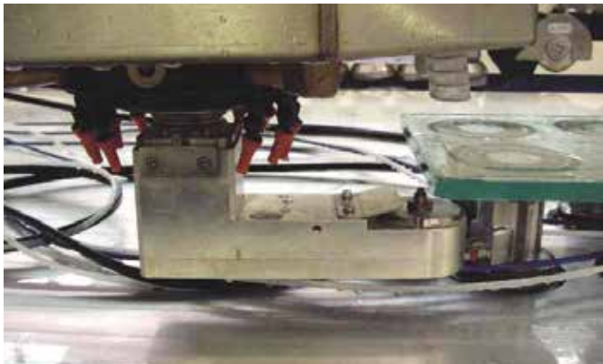
UNITE DE PERCAGE AVEC TRANSMISSION ANGULAIRE En utilisant ce dispositif, il est possible de percer de fines plaques de verre sans écaillage.
